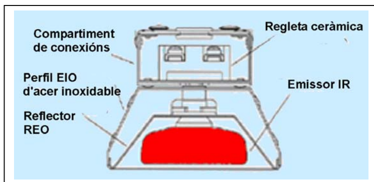
Secció d'un conjunt EBI
