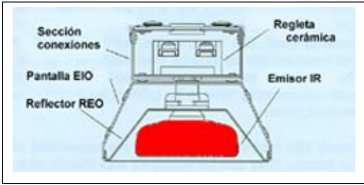
Sección de un conjunto EBI
