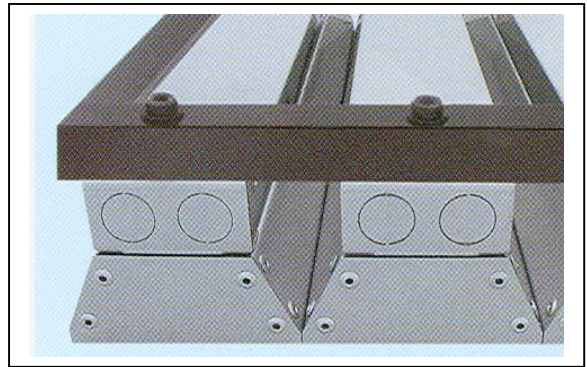
Ensamblaje de varios EBI, para construir un panel
